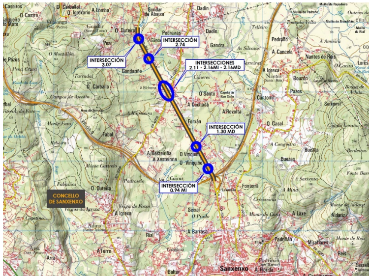
Planta das interseccións nos puntos quilométricos 2+110 e 2+160
