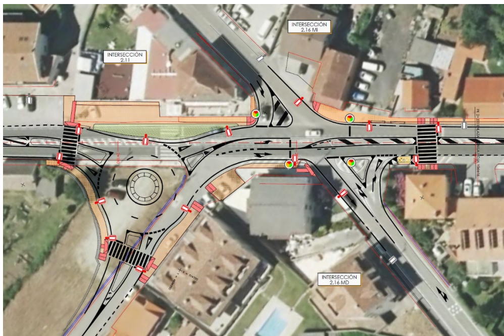
Planta das interseccións nos puntos quilométricos 2+110 e 2+160
